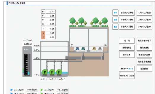
設備図
