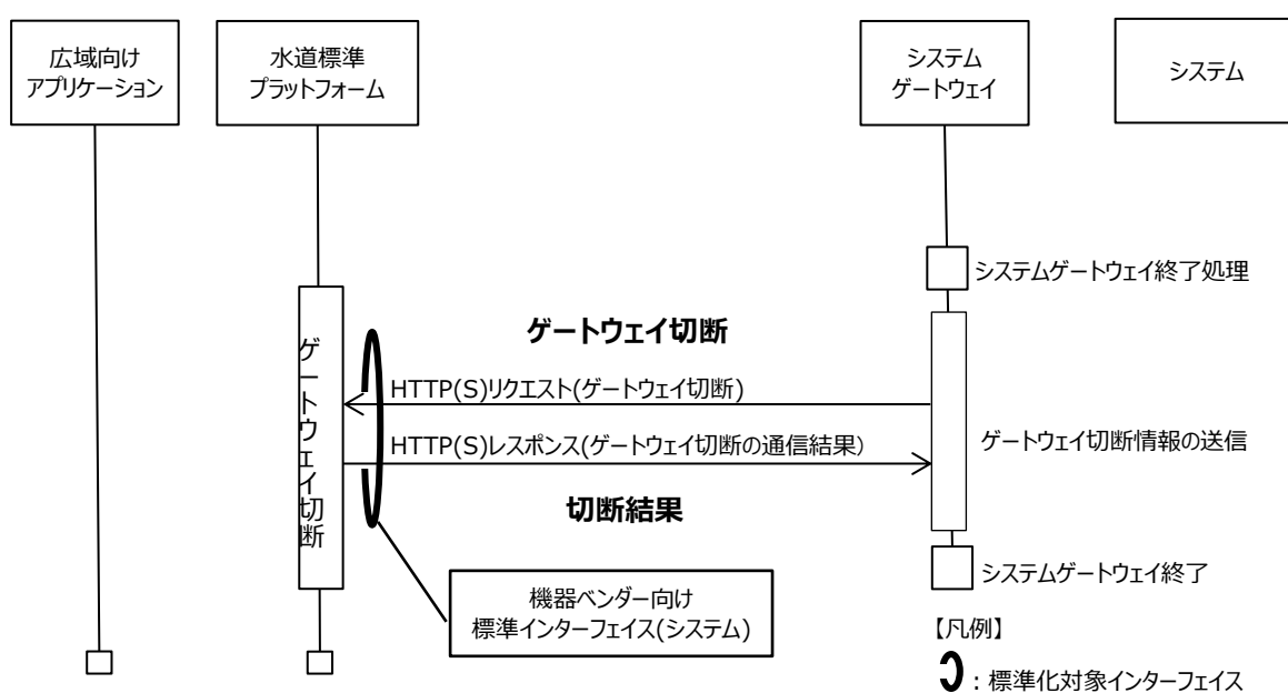
図 4-2: ゲートウェイ切断の詳細フロー
