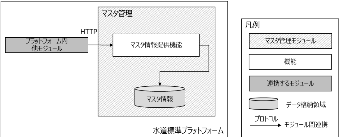
図 8-1 : マスタ管理 機能(モジュール)構成
